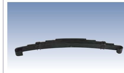
SL082 スプリング 5リーフ フック サイズ:69×16×4×63cm(長さ×高さ×幅×取付ピッチ) 品番 4610048 (1ヶ)¥12,915 ¥12,300
