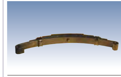
SL081 スプリング 5リーフ フック サイズ:58×15×4×54cm(長さ×高さ×幅×取付ピッチ) 品番 4610072 (1ヶ)¥10,920 ¥10,400
