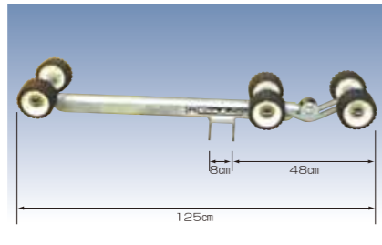
SL065 6ローラー ローラーアーム 2x3 品番 6220400 (1本)¥51,660 ¥49,200
