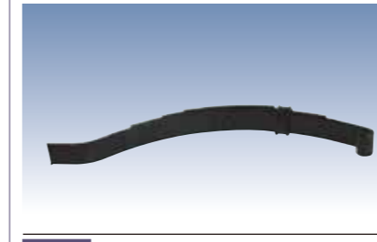
SL080 スプリング 4リーフ スリッパ サイズ:58×15×4×54cm(長さ×高さ×幅×取付ピッチ) 品番 4610010 (1ヶ)¥8,820 ¥8,400
