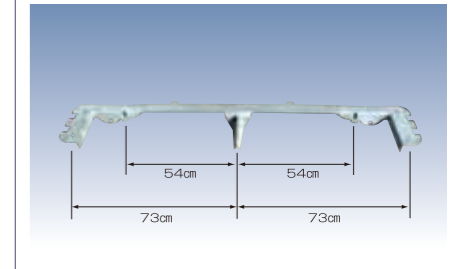
SL125 スプリング BRKT9インチTANDEM(40T/46T) 品番 6616300 (1ヶ)¥27,090 ¥25,800
